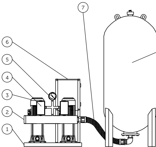
GRUPO DE PRESIÓN DOBLE HIDRONEUMÁTICO
