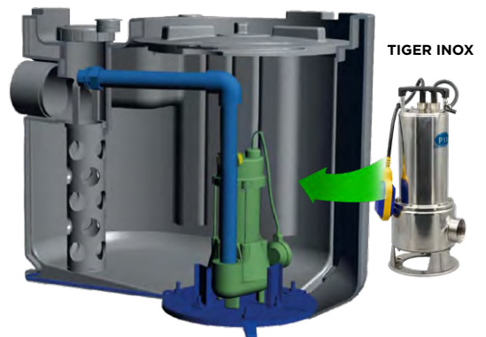
AQUATANK 100
