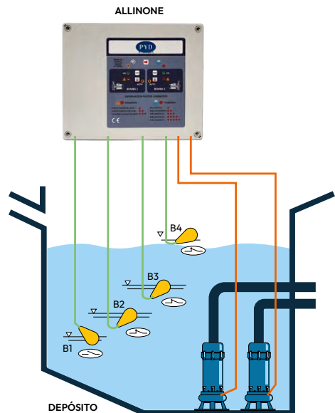
ELECTROBOMBAS DE AGUAS RESIDUALES CON BOYAS
