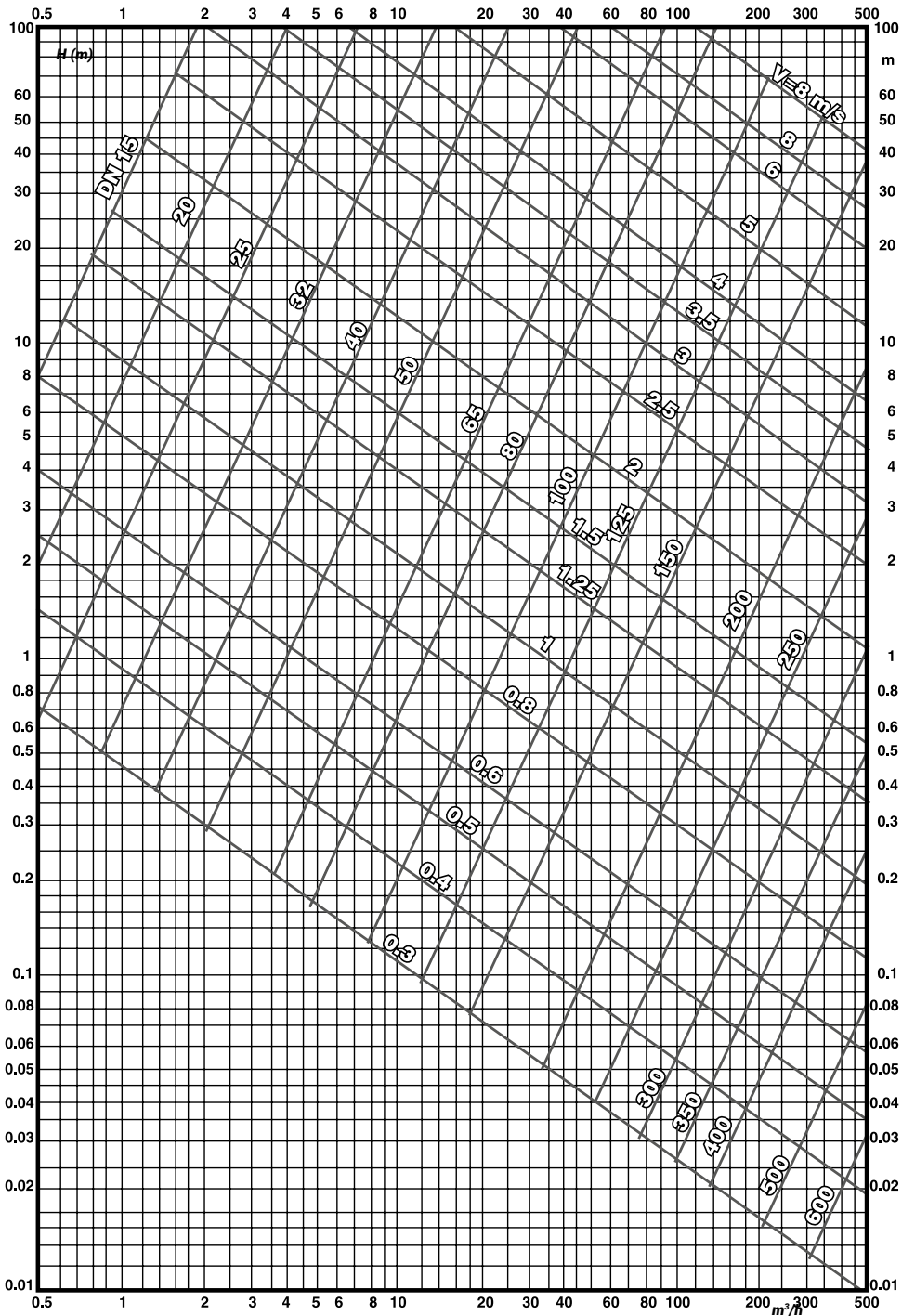
Pérdida de carga Hv por cada 100 metros de tubería
